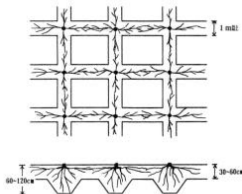
図－6－3 格子状客土
